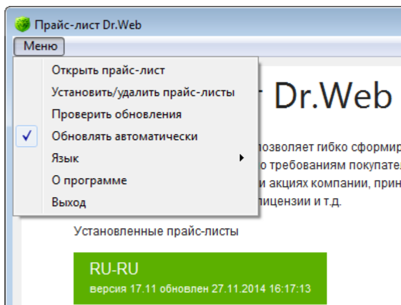
Рисунок 2. Меню программы
