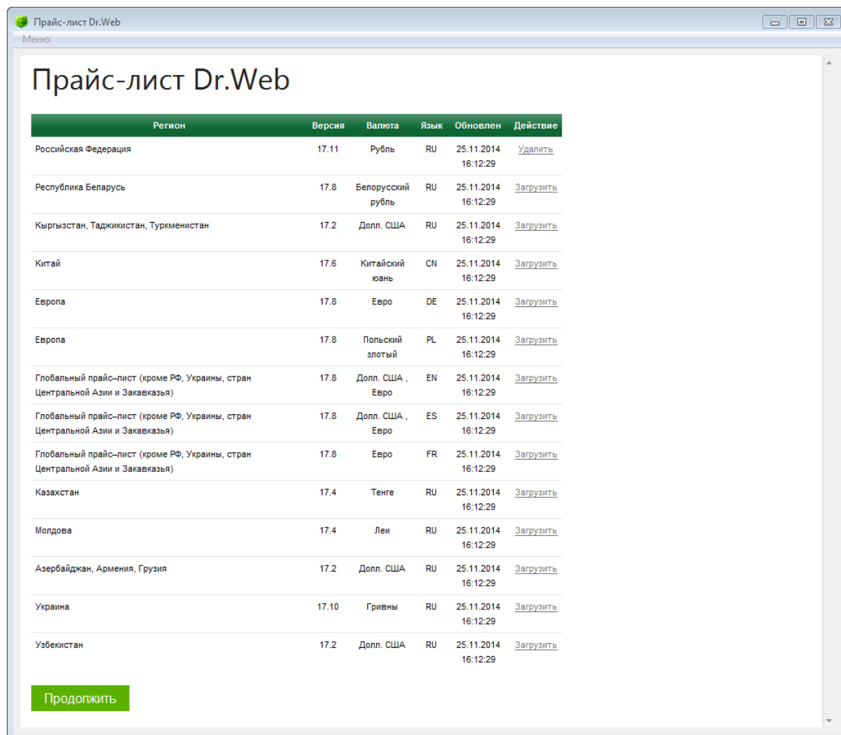
Рисунок 1. Управление прайс-листами
