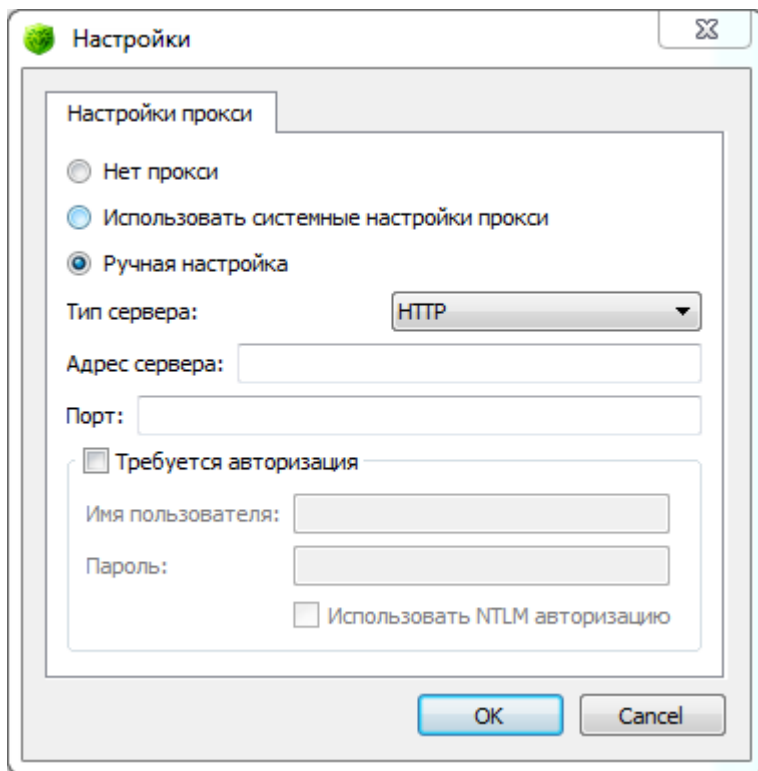
Рисунок 3. Настройка прокси-сервера
